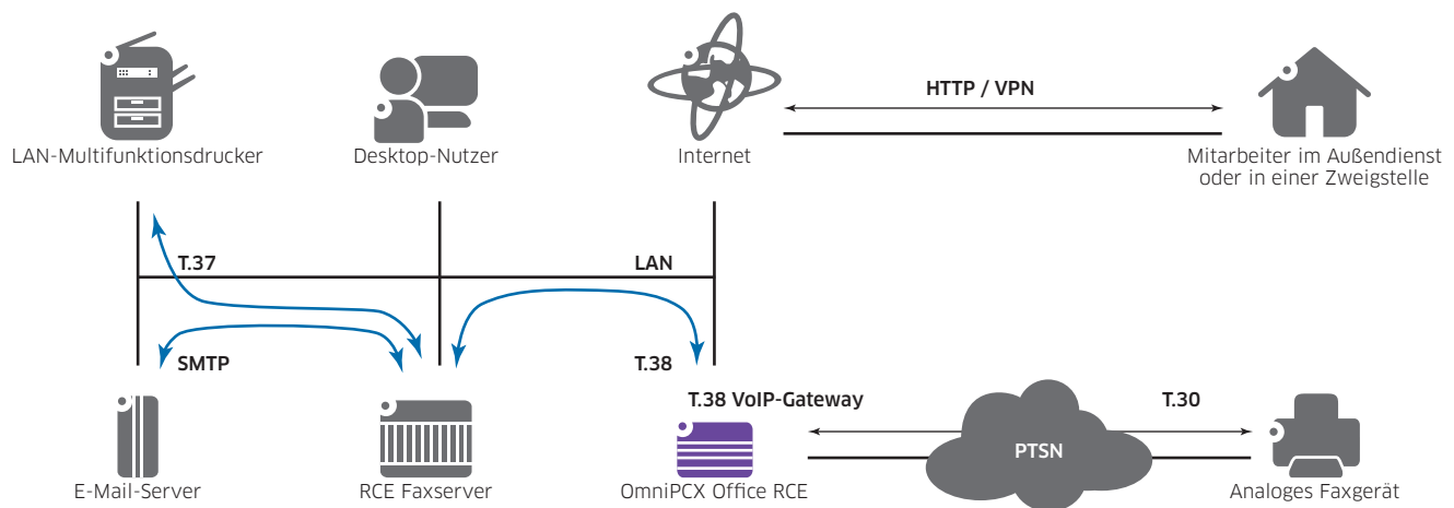
Abbildung 1. Die Alcatel-Lucent OmniPCX Office RCE Fax-Server-Topologie
